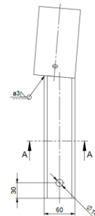
DETALJ C (1 : 1)
