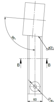
DETALJ C (1 : 1)
