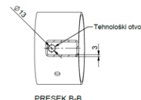
PRESEK B-B
