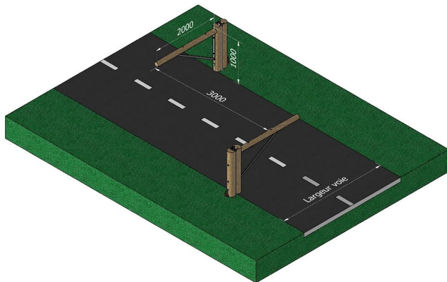
Position fermée – ensemble posé en quinconce
