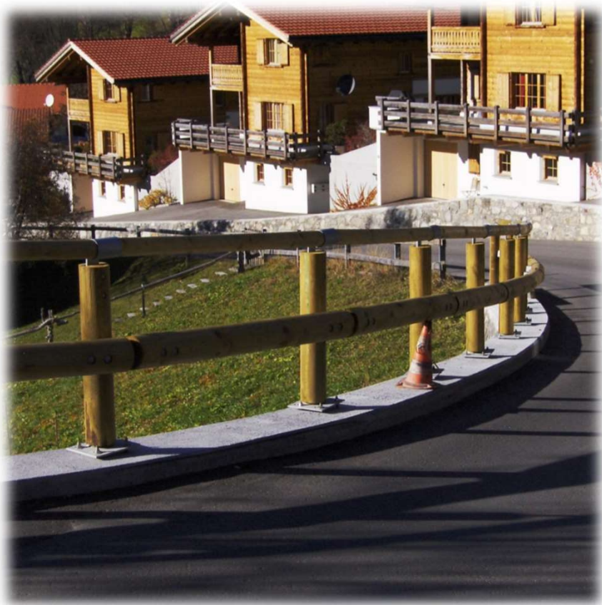
SOLOBOIS avec réhausse main courante à l'aplomb et habillages rallongés
