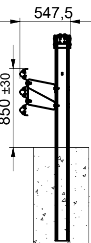
PRESEK A-A
