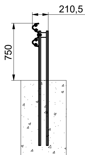
PRESEK A-A
