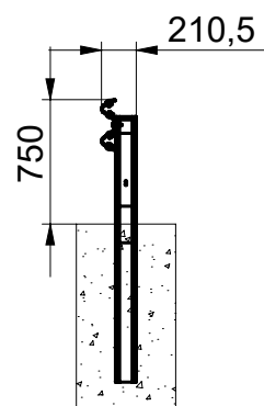
PRESEK A-A
