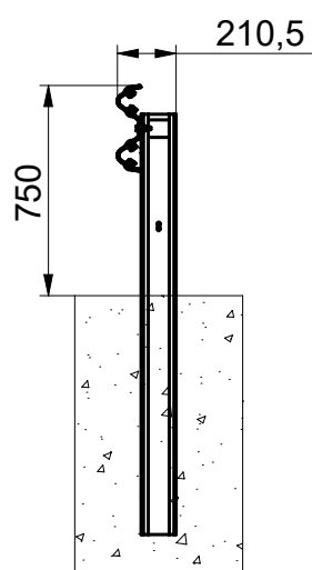
PRESEK A-A
