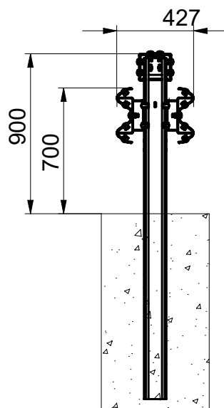
PRESEK A-A
