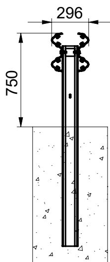
PRESEK A-A
