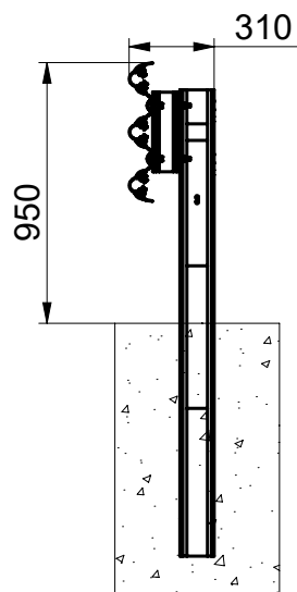
PRESEK A-A
