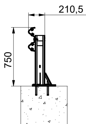
PRESEK A-A
