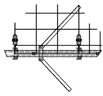
Detalj B ( 1 : 10 )
