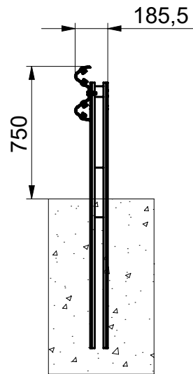
PRESEK A-A
