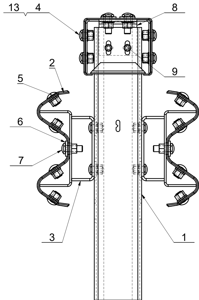
DETALJ X (1 : 5)
