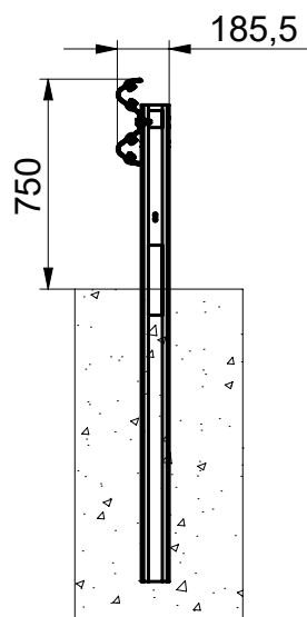
PRESEK A-A
