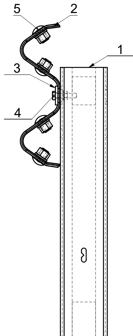
DETALJ X (1 : 5)
