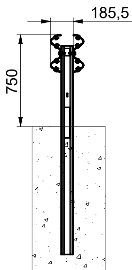
PRESEK A-A
