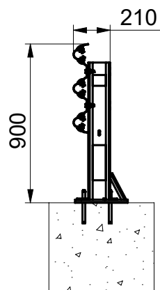
PRESEK A-A
