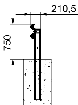
PRESEK A-A
