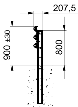
PRESEK A-A
